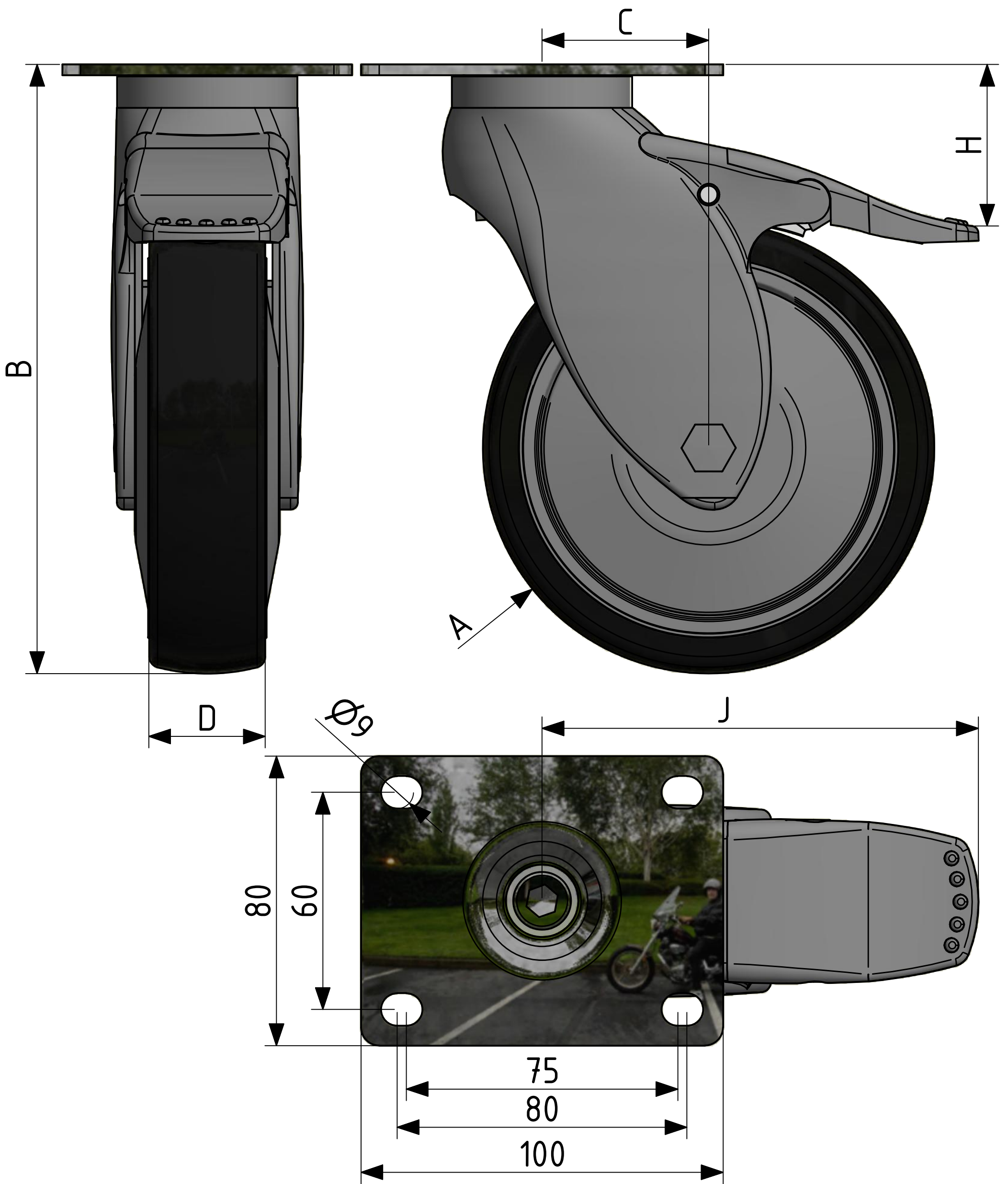
Masstabelle KSF mit Plattenbefestigung
