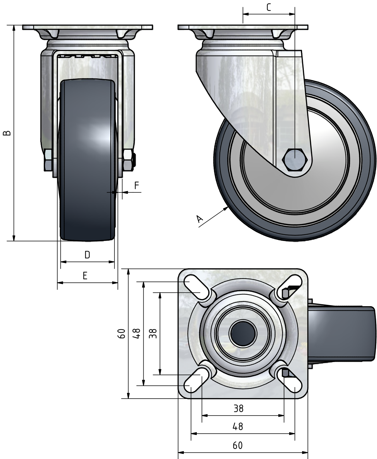
Maßtabelle NGML-31C-P60
